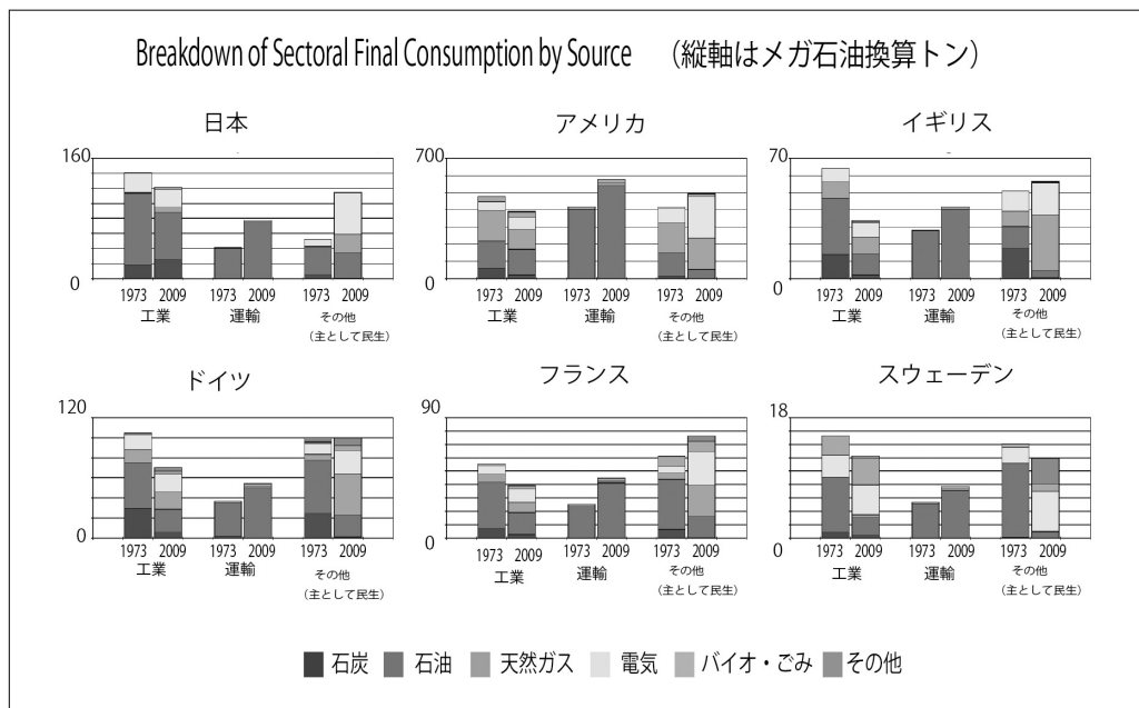
図ー1 1973年と2009年における最終エネルギー消費の6先進諸国についての比較。データはIEA (International Energy Agency) による。日本では民生部門が倍に急増していることと、石油、電気の消費が多くエネルギーの多様性が少ないことが見て取れる。
